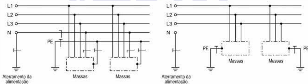
Figura 4 — Esquema TT
